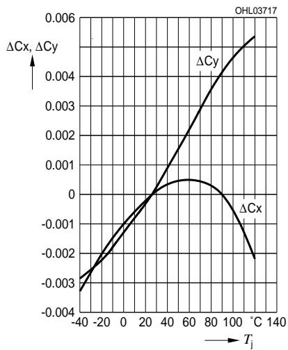
Chromaticity Coordinate Shift 6) page 25 Farbortverschiebung 6) Seite 25 C_x, C_y = f(T_j); I_F = 30\text{ mA}
