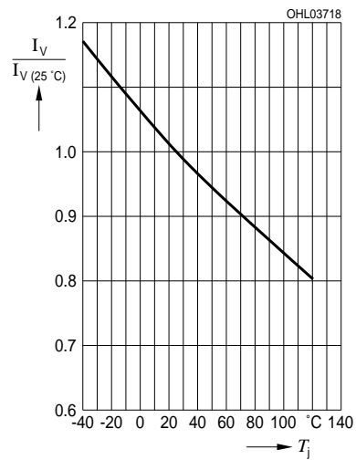
Relative Luminous Intensity 6) page 25 Relative Lichtstärke 6) Seite 25 I_V/I_V(25^\circ\text{C}) = f(T_j); I_F = 30\text{ mA}
