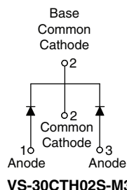
D 2 PAK (TO-263AB)
