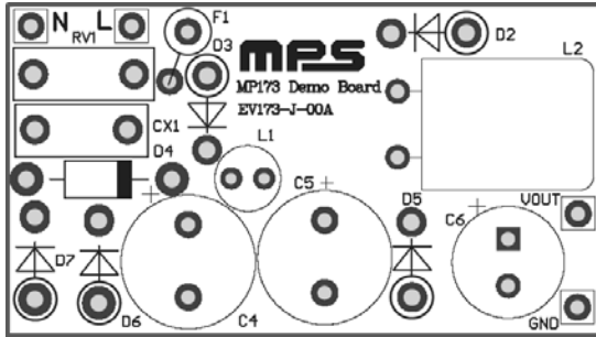
Top layer
