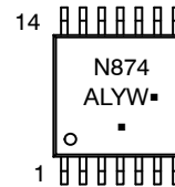
TSSOP-14 WB CASE 948G
