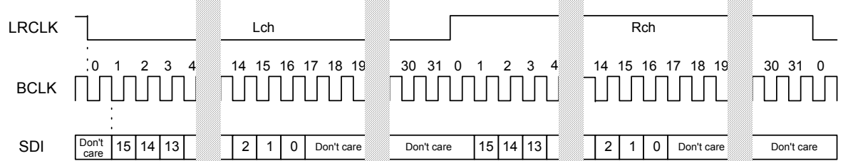
Fig.29 AUDIO I/F Format (BU7893GU)
