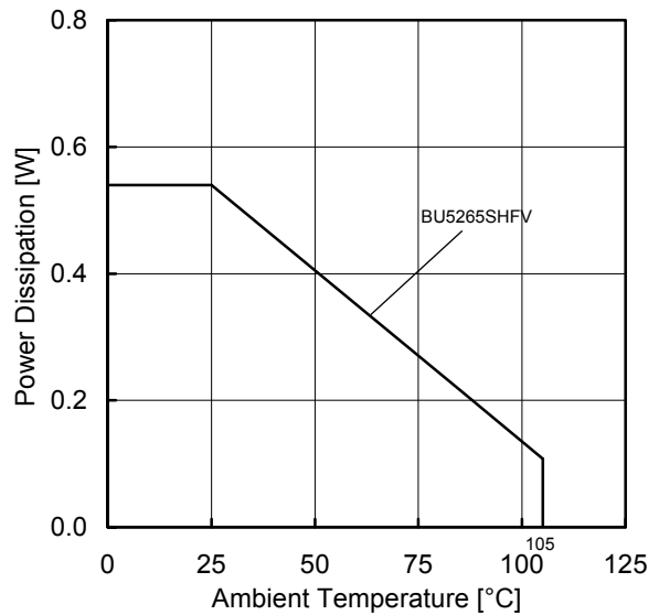
(d) BU5265SHFV
