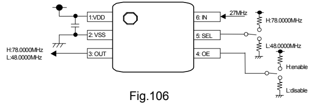
(BU7325HFV)
