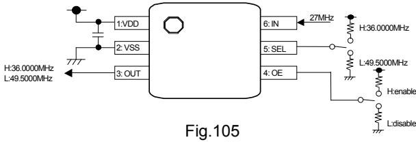
(BU7322HFV)
