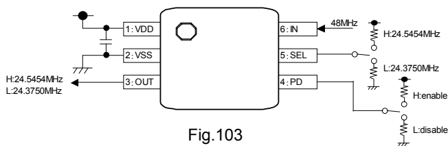
(BU7322HFV)
