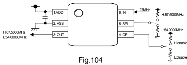
(BU7325HFV)
