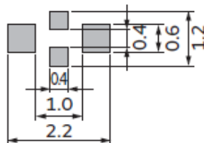
NFM18CC/18PC
