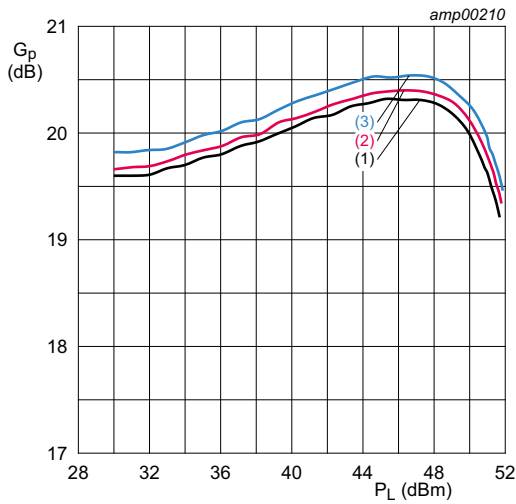
V_{DS} = 28\text{ V}; I_{Dq} = 1600\text{ mA}. (1) f = 2115\text{ MHz} (2) f = 2140\text{ MHz} (3) f = 2165\text{ MHz}
