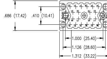
20 PIN RECEPTACLE
