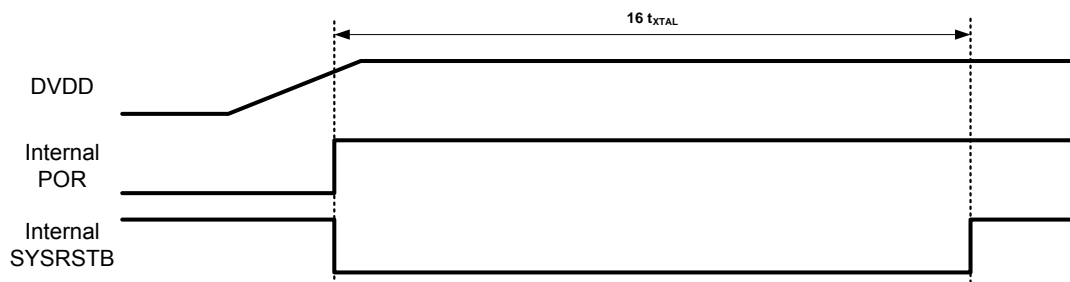
Figure 32. POR Timing
