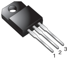
ITO-220AB
