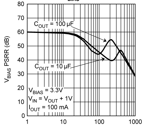
V_{BIAS} PSRR
