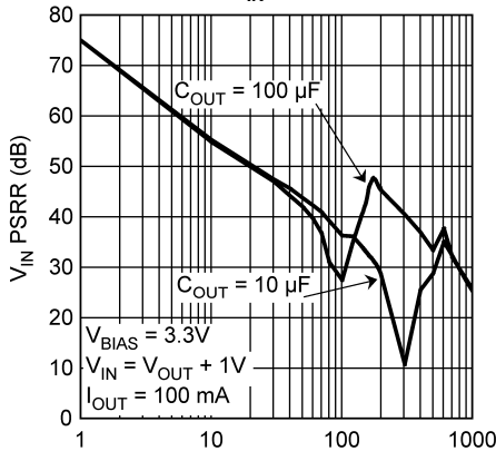
V_{IN} PSRR
