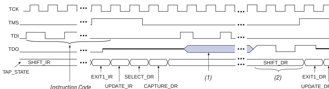
Figure 13-9. SAMPLE/PRELOAD Shift Data Register Waveforms
