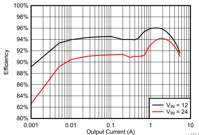
LMS3655-Q1 Efficiency: V_{\text{OUT}} = 5\text{ V}
