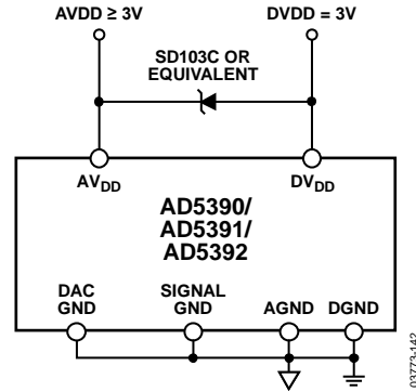
Figure 42. DV DD first followed by AV DD
