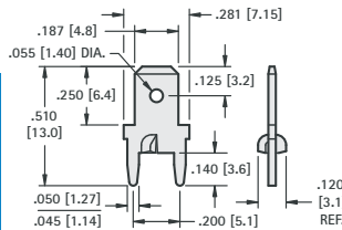
.187 (4.8) TAB
