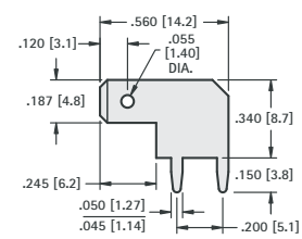
.187 (4.8) TAB
