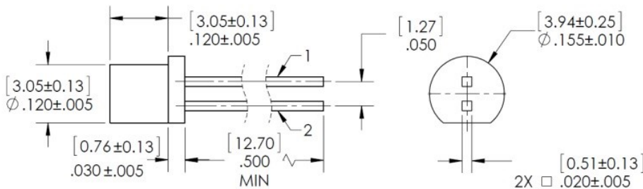
OP506
