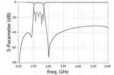
RFBPF1109B201T
