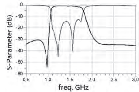
RFBPF1109B101T
