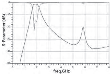
RFBPF1109B301T
