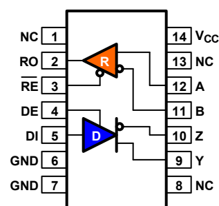
ISL3150E, ISL3153E, ISL3156E (14 Ld SOIC) Top View
