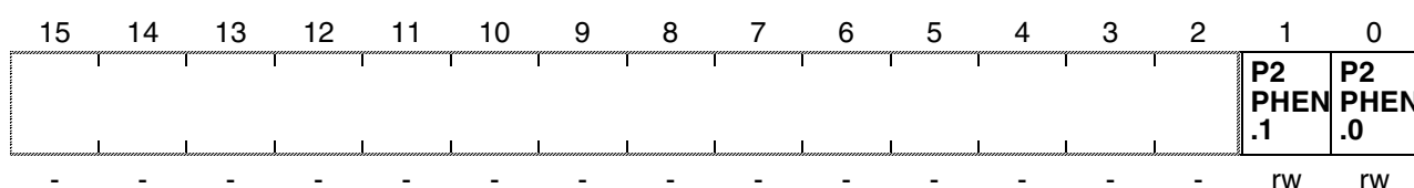
P2PHEN (FE7C H / 3E H ) SFR Reset Value: - - 00 H
