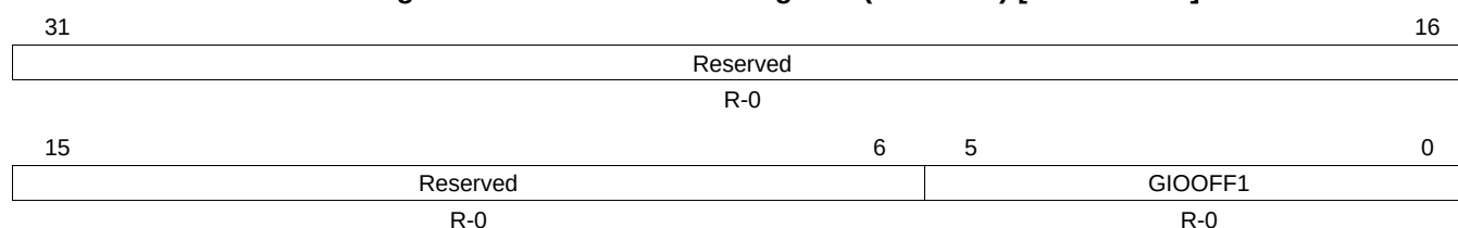
Figure 22-13. GIO Offset 1 Register (GIOOFF1) [offset = 24h]
