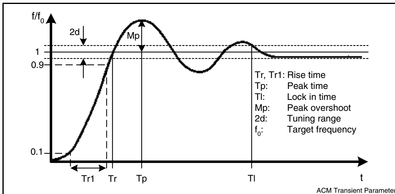
Figure 20 Transient Parameters
