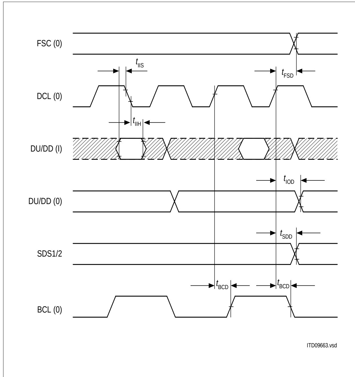
Figure 85 IOM ® Timing
