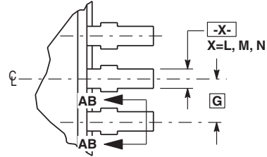
VIEW Y
