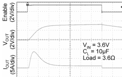
TIME (4 \mu s /div)
