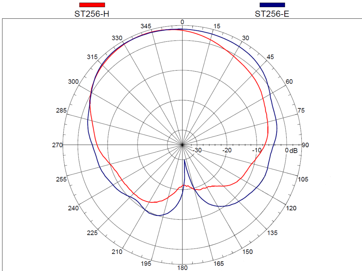
Red Line : H-plane ; Blue Line : E-plane
