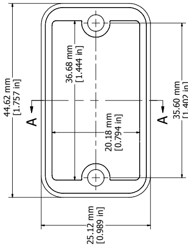
OPEN BEZEL
