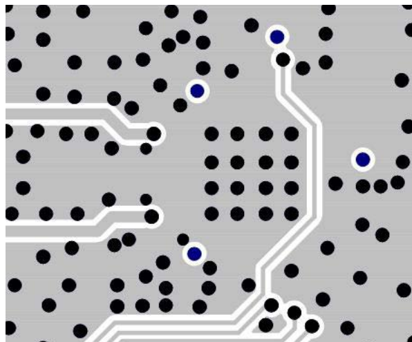
Inner Layer 4
