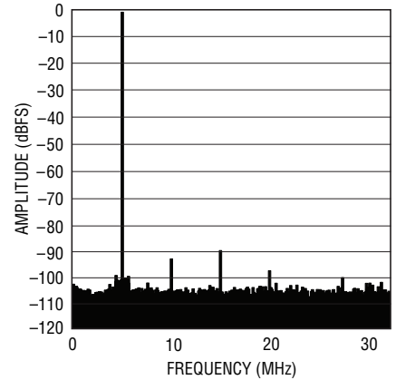
LTC2265-14: 8k Point FFT, f_{IN} = 5\text{MHz} , -1\text{dBFS} , 65\text{Mpsps}
