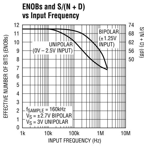
LTC1282 • TPC05
