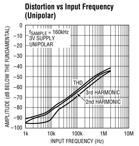
LTC1282 • TPC06
