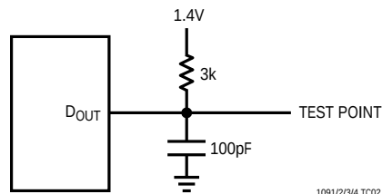
Load Circuit for t_{dO} , t_r , t_f
