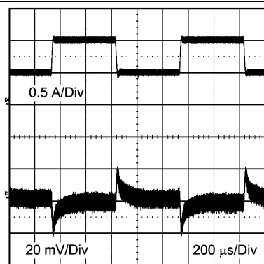
12 V_{IN} 3.3 V_O 0.6-A to 1-A Step
