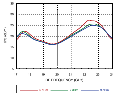
Input IP3, USB vs. LO Drive
