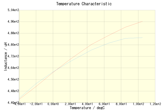
CLF6045T-471M-CA(DC = 0A)
