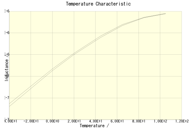
CLF12555T-1R0N-CA(DC = 0A)
