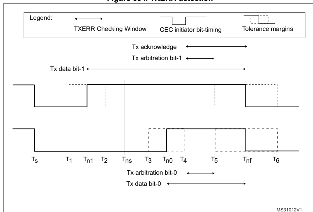
Figure 534. TXERR detection
