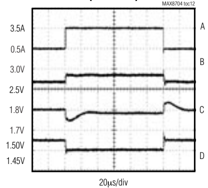
3A LOAD TRANSIENT (FDS6570A)
