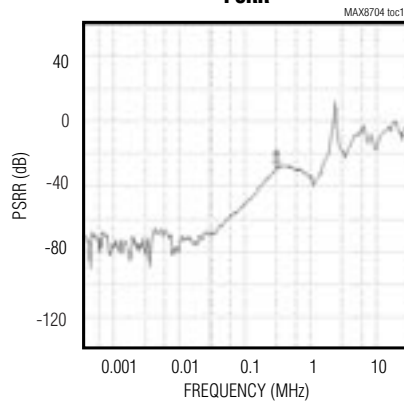
PSRR
