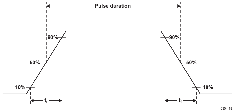
Figure 6-62. UART IrDA Pulse Parameters
