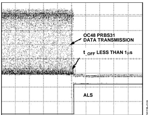
Figure 17. ALS Assert Time, 5\ \mu\text{s}/\text{DIV}
