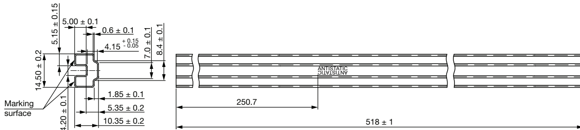
Fig. 16 - DIP-6
