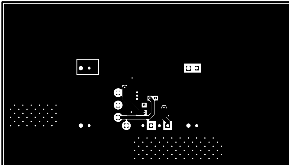
Figure 25. Bottom Layer
