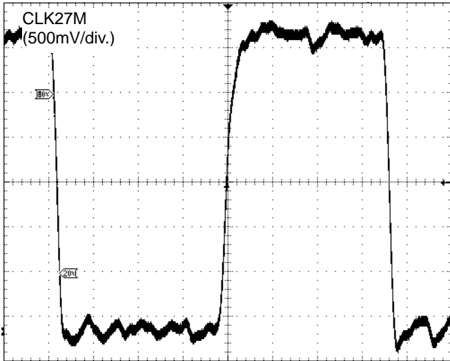
TIME (5nsec/div.)
