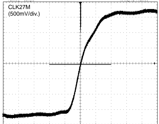
TIME (1nsec/div.)
