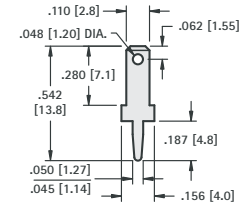
.110 (2.8) TAB
