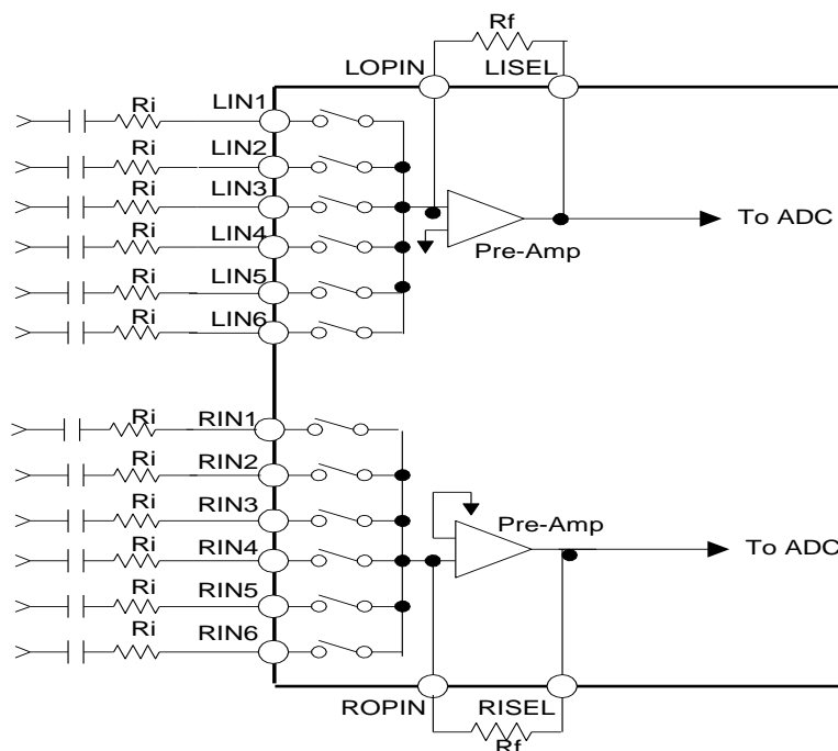
Figure 21. Input ATT
