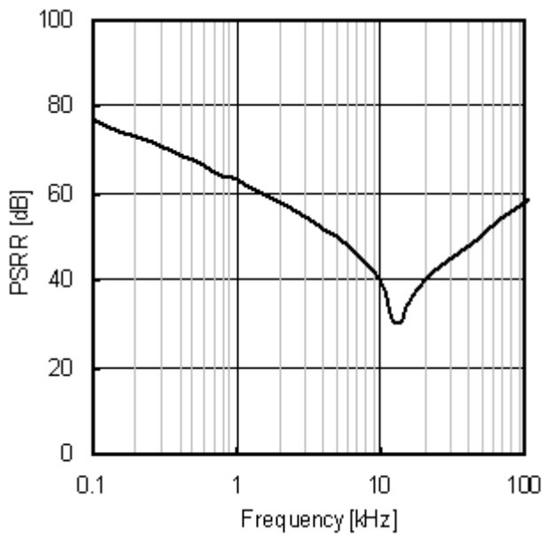
Fig.33 PSRR(Io=0A)
