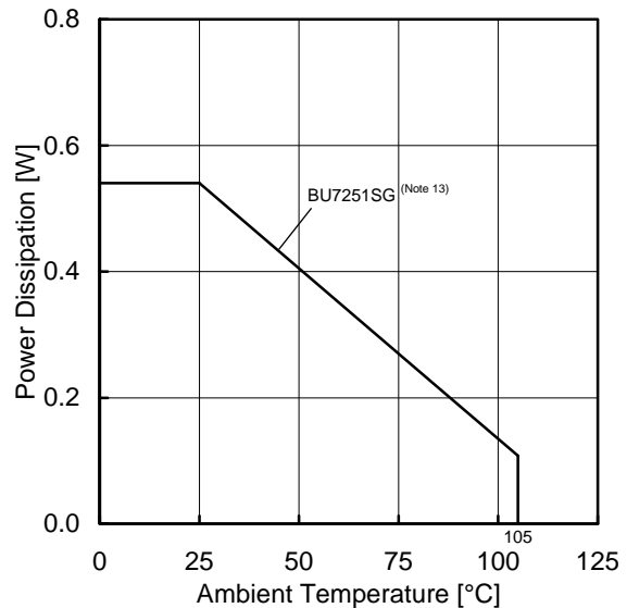
(d) BU7251SG
