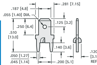
.187 (4.8) TAB
