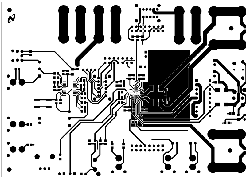
Figure 6-2. Top Layer
